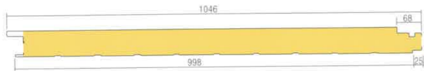
▶ 그라스울판넬 형상
