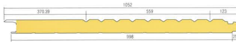
▶ 그라스울판넬 형상
