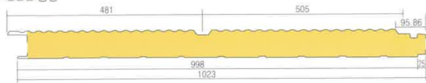
▶ 그라스울판넬 형상
