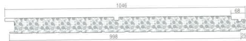
▶ 난연 EPS판넬 형상
