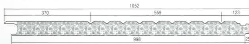
▶ 난연 EPS판넬 형상
