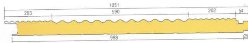
▶ 그라스울판넬 형상
