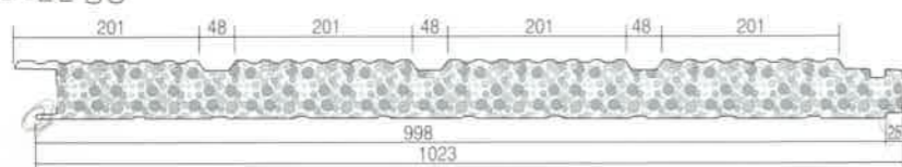
▶ 난연 EPS판넬 형상
