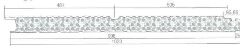
▶ 난연 EPS판넬 형상
