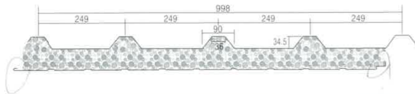
▶ 난연 EPS판넬 형상
