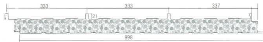
▶ 난연 EPS판넬 형상
