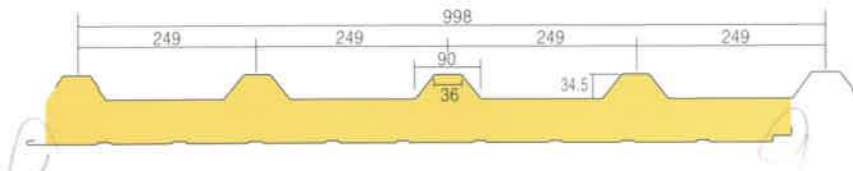
▶ 난연 EPS판넬 형상
